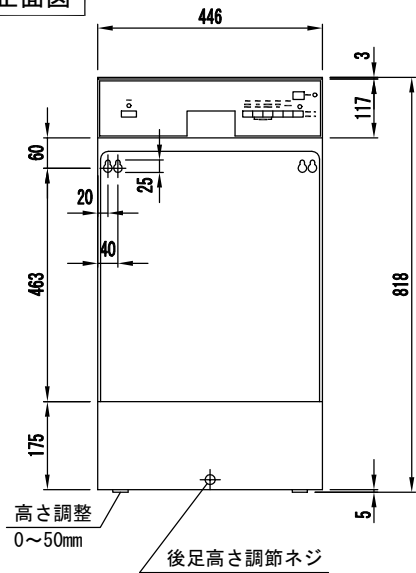
正面図
