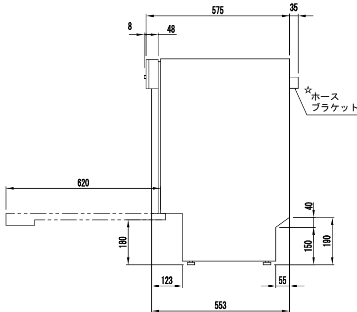
右側面図
